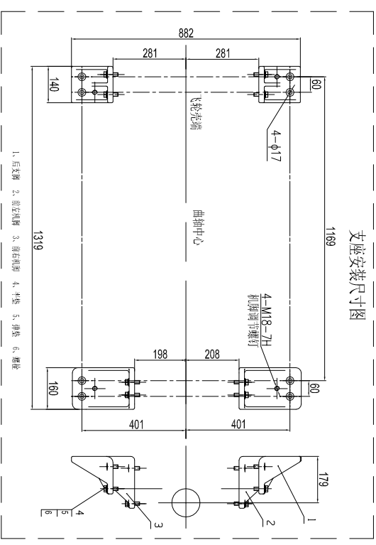
YC6T系列船机外形安装图(双孔支脚)
